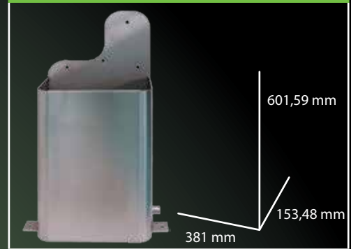
PS001 - Cestello Portaspazzola/Basket for brush holder device
